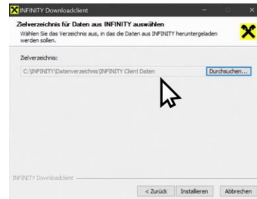
Schritt 2: Datenverzeichnis
