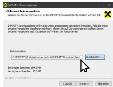
Schritt 1: Installationsverzeichnis
